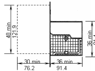
(d) Clear Floor Space at Shower
